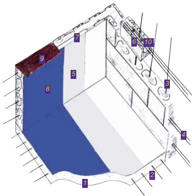
Semelle en acier pour bloc coffrant
